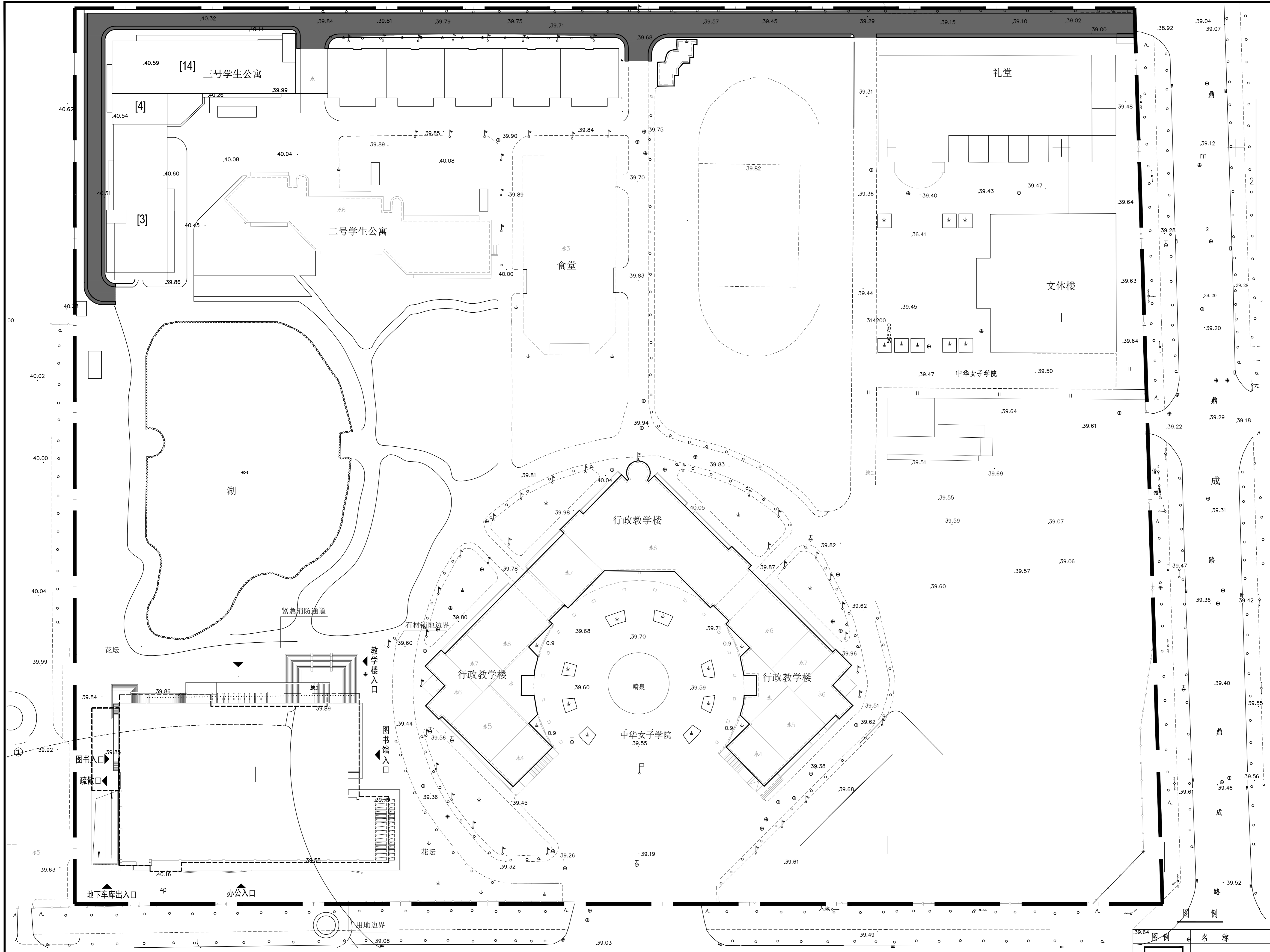
现状总平面图 1:500
